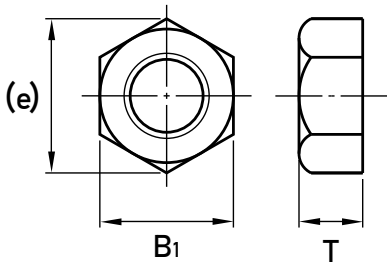
Nut parameters
